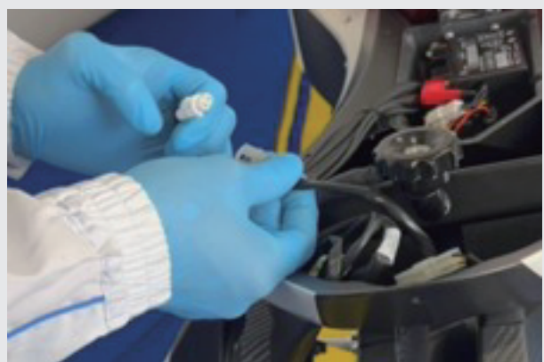
5.灰色のカプラーを取り外します
